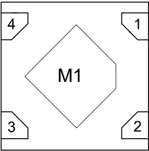
图 3 底视图
